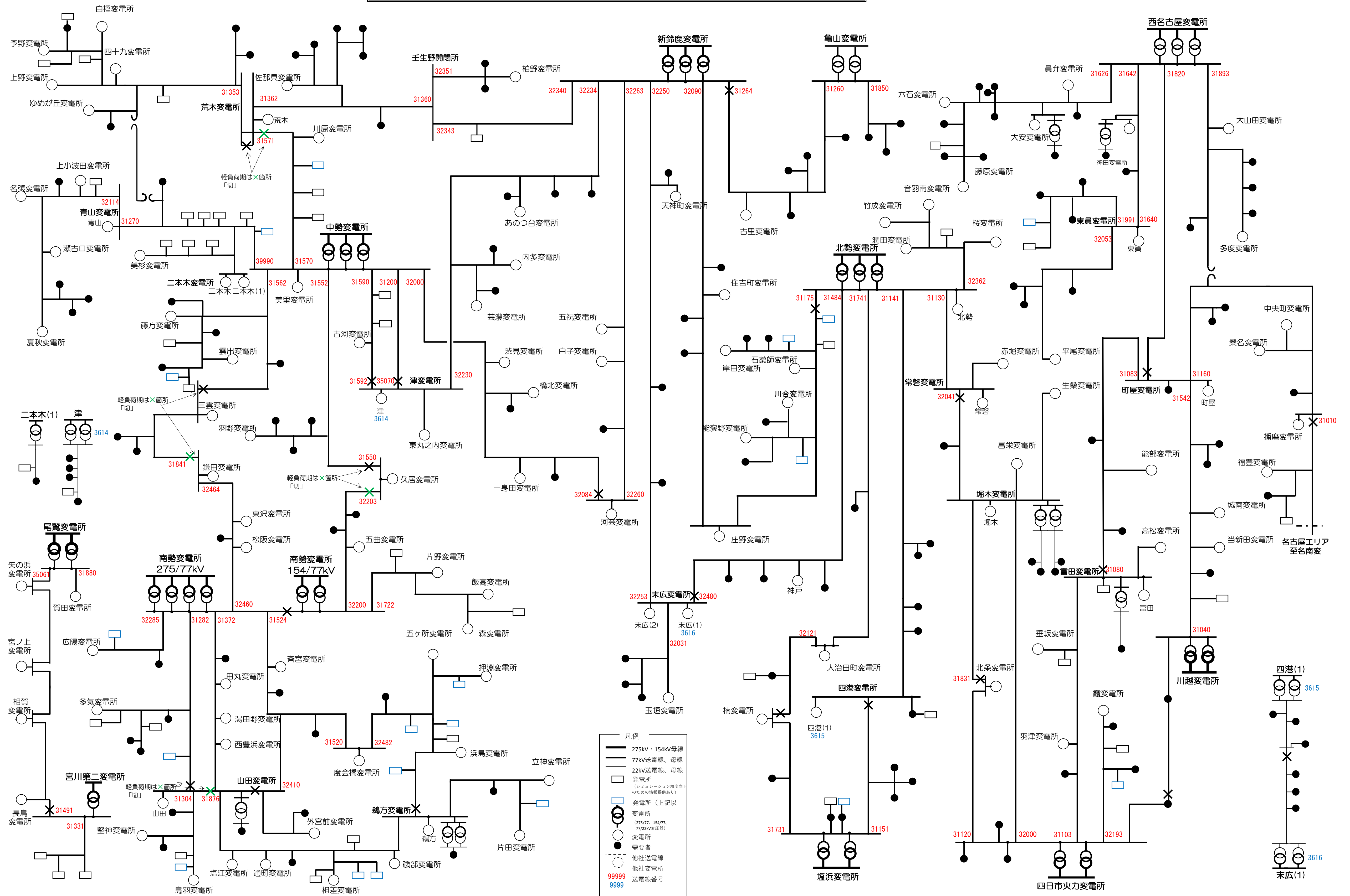
77kV以下系統構成図（三重県）（2025年度 基本系統）
