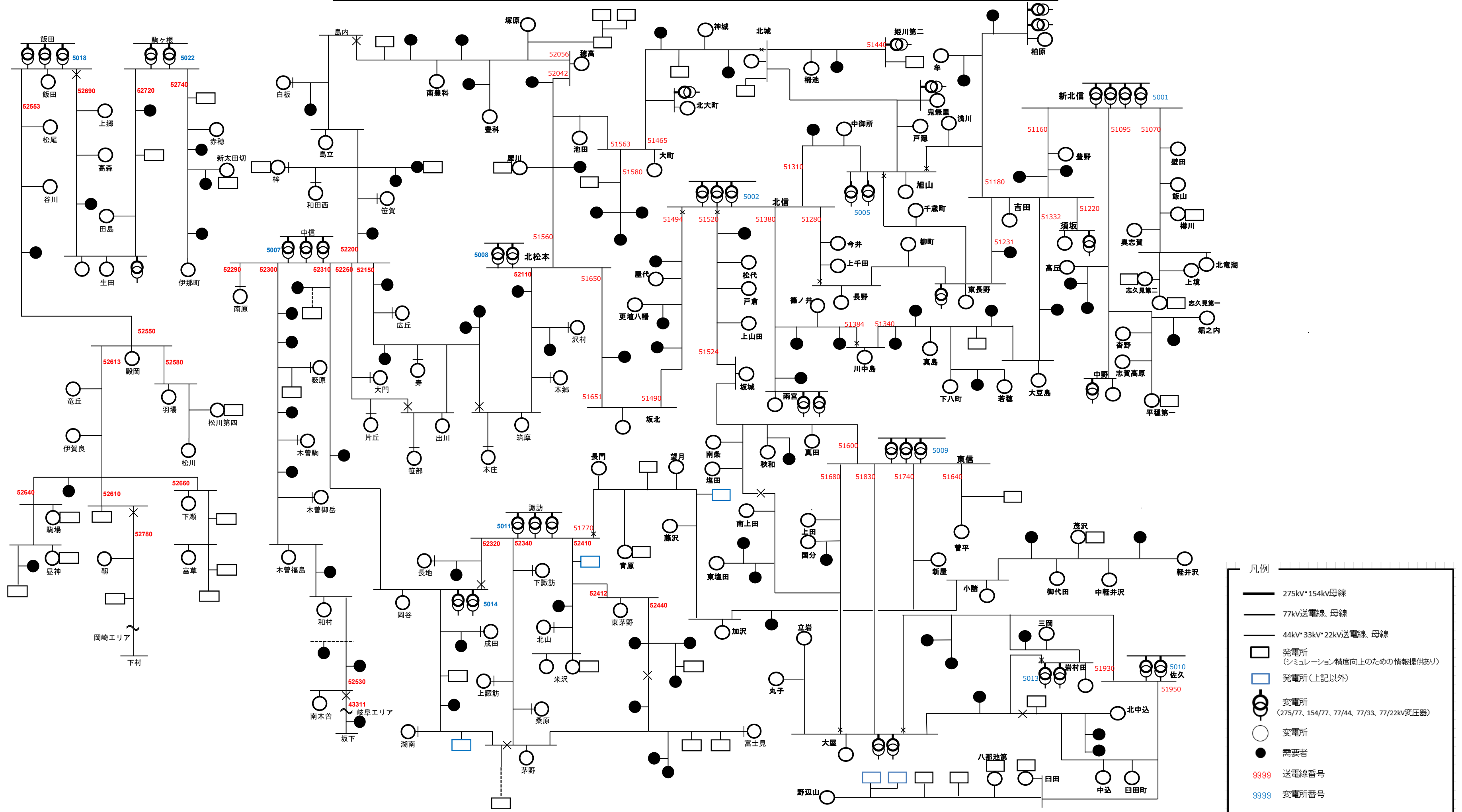
77kV系統構成図（長野県）（2025年度 基本系統）
