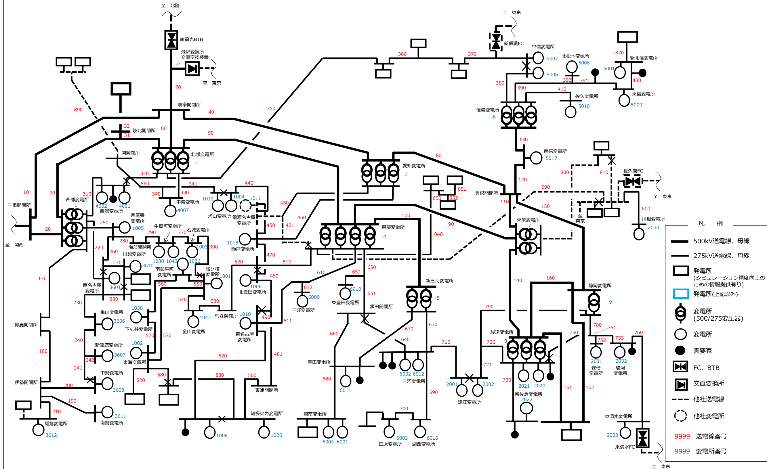
500kV・275kV系統構成図 (2025年度 基本系統)
