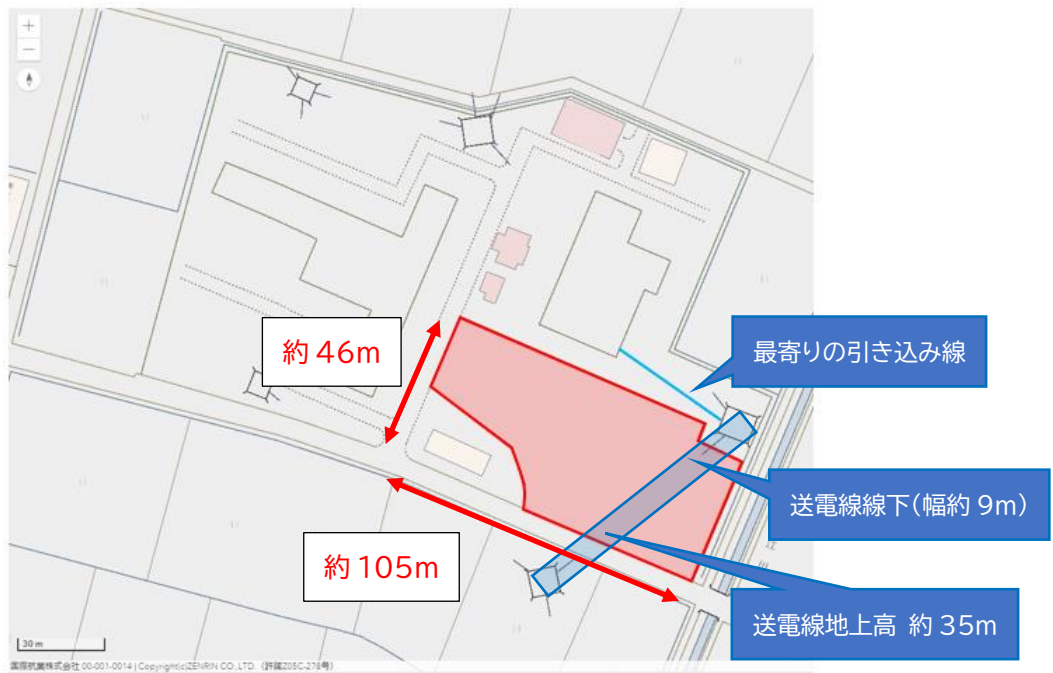
南大垣変電所 構内
