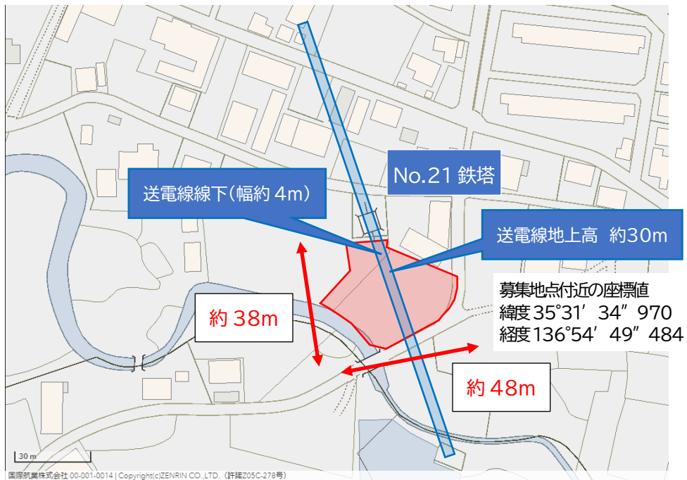
77kV 関美濃線 No.21 鉄塔余剰地
